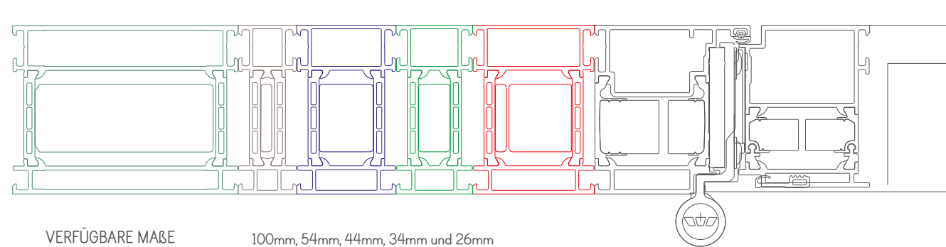
ALU-VERBREITERUNGEN SEITLICH UND OBERHALB ALU-LATERAL AND UPPER EXPANSION
