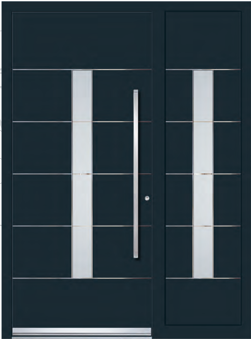
Modell ZU 48E Farbe RAL 7016 MATT Verglasung DPH Intarsien POLIERT Griff KPR 115h Rosette RMM Designsockel JZP 50 Seitenteil rechts ZU 48E
